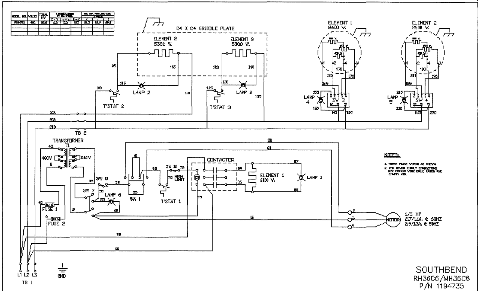
SE36A-TTB WIRING DIAGRAM 480V
