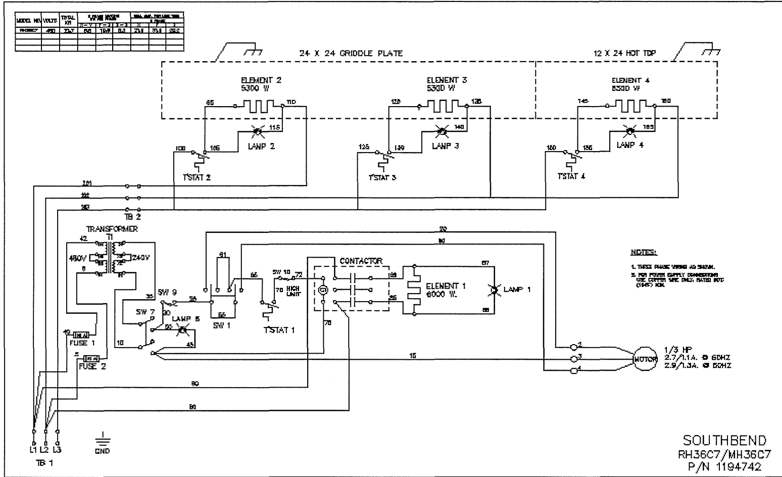
SE36A-TTH WIRING DIAGRAM 480V
