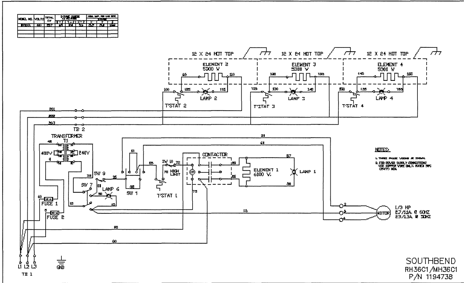
SE36A-HHH WIRING DIAGRAM 480V
