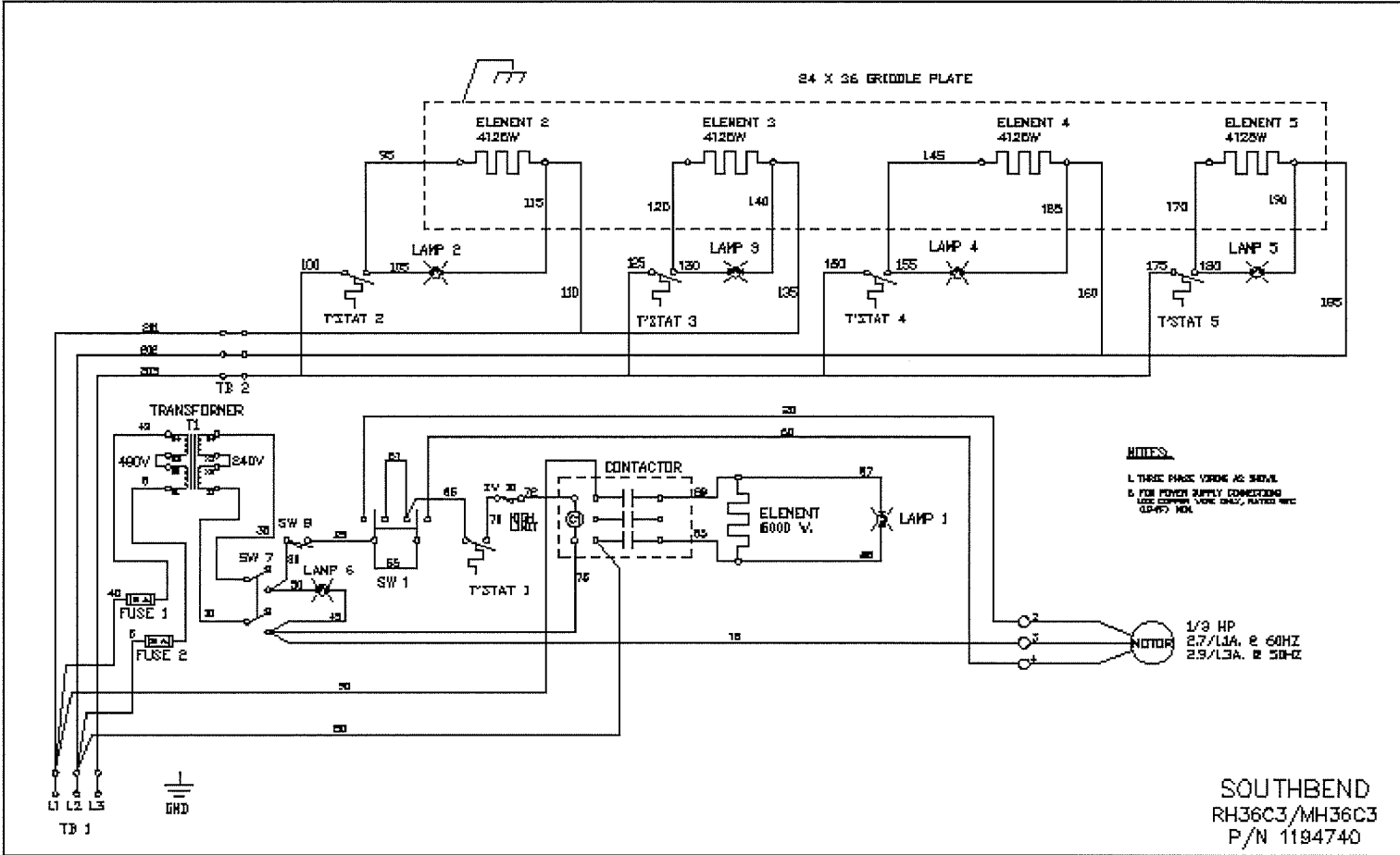
SE36A-TTT WIRING DIAGRAM 480V
