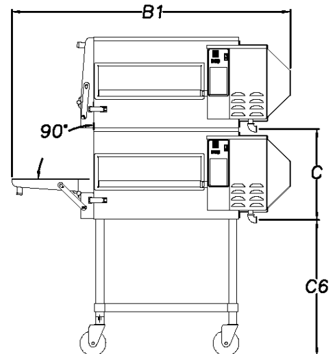
VUE D'EXTRÉMITÉ DOUBLE PILE
